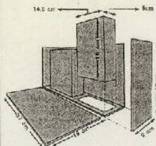
Esquema del molde
